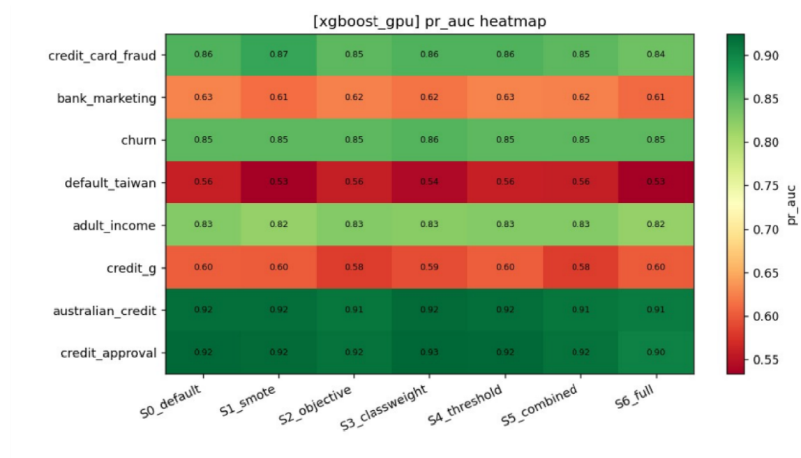
Fig 4.10: PR-AUC Heatmap (XGBoost-GPU)
